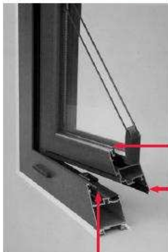
A fermavetro B battuta centrale C battuta interna
